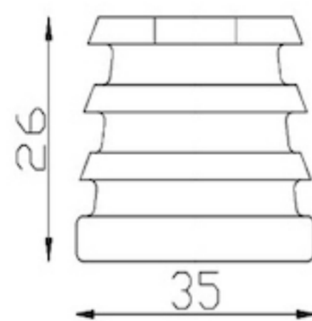
Bouchon percé M10
