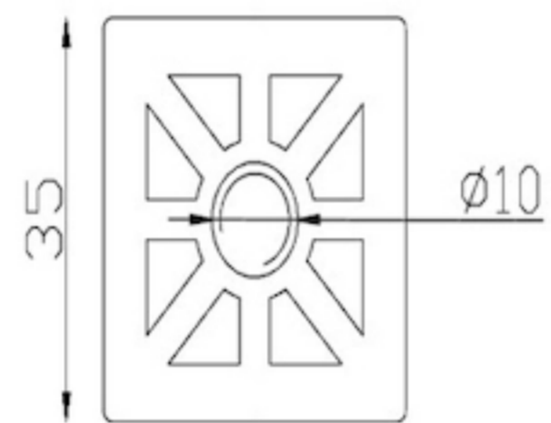
Bouchon percé M10
